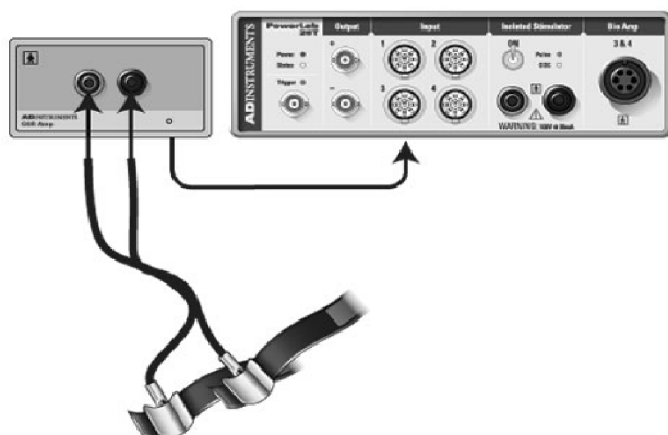
Obrázek 17. Schématické znázornění měřicího přístroje ADInstrument Power Lab spolu se zesilovačem ML 116 GRS Amp a s elektrodami. Dostupné z www.adinstrument.com .
